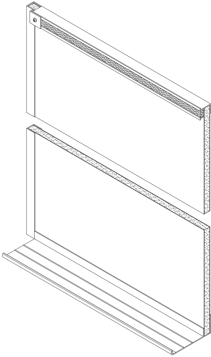
SECTIONAL ISOMETRIC SCALE: 3" = 1'-0"
