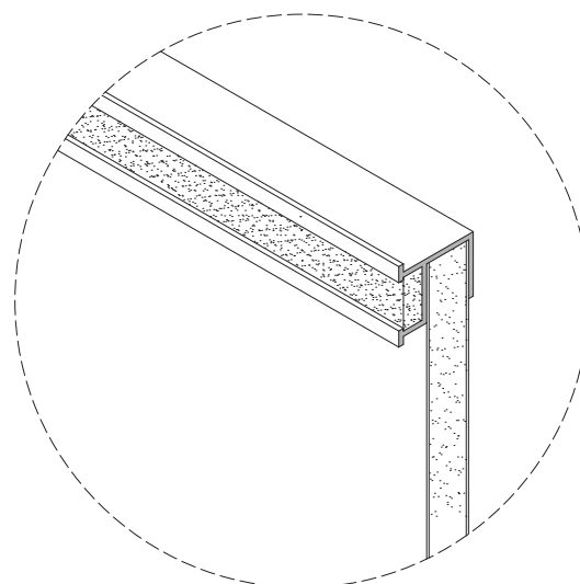
SCREW-ON MAPRAIL SCALE: 6" = 1'-0"
