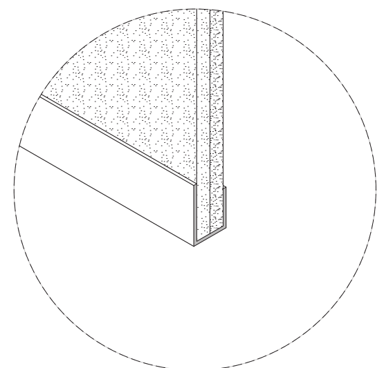
SCREW-ON MITERED TRIM SCALE: 6" = 1'-0"
