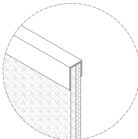
SCREW-ON MITERED TRIM SCALE: 6" = 1'-0"
